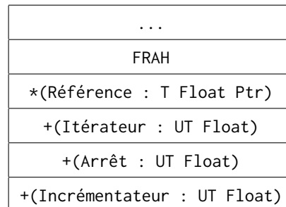
FIGURE 11 – Bloc d'activation de la boucle for
