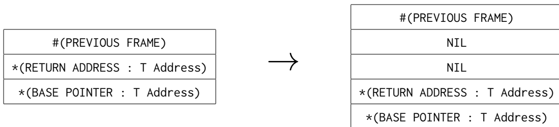
FIGURE 12 – Effet de _nil_fill sur la pile
