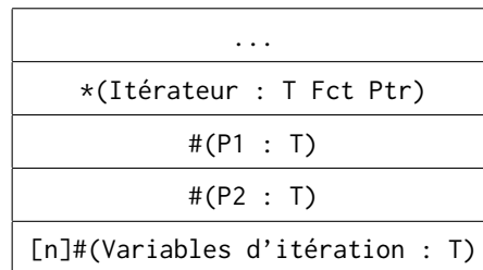
FIGURE 10 – Bloc d'activation de la boucle for .. in
