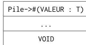
FIGURE 7 – Format d'une pile
